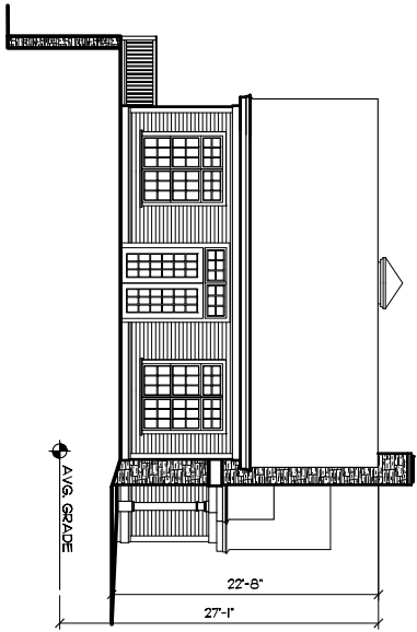
LEFT ELEVATION Scale: 1/8" = 1'-0"
